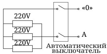
Рисунок 9. Схемы соединения блока ТЭН
